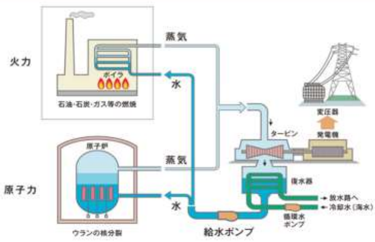
図1. 火力発電と原子力発電の違い
