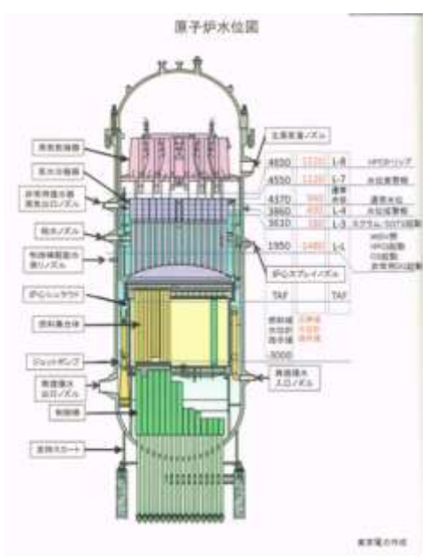
図2. 原子炉の中には約2年分の燃料が予め挿入されている（黄色の部分）
